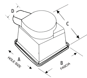
Dimensions - WhisperVent 100
